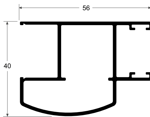
2529R Pierna Reforzada TP 0.809 kg/m
