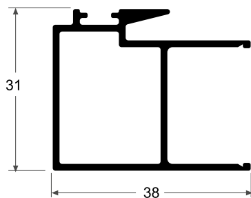
2519 Traslapo TP 0.517 kg/m
