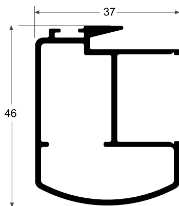
2530R Traslapo Reforzado TP 0.729 kg/m
