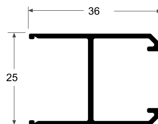
2550 Pierna Hoja Fija TP 0.378 kg/m
