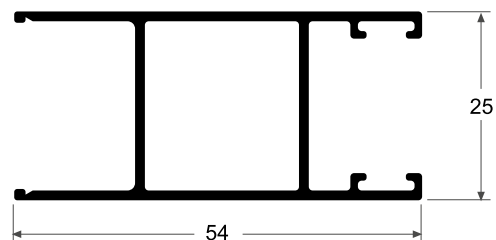
2517 Pierna Abierta TP 0.578 kg/m
