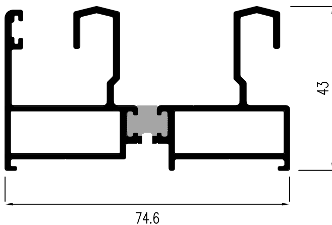
3324R Riel RPT 1.415 kg/m
