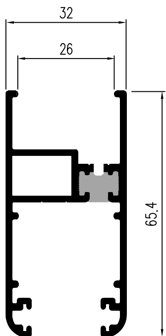
3308R Hoja TP RPT 1.036 kg/m
