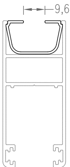
S284 Adaptador Monolitico 0.160 kg/m
