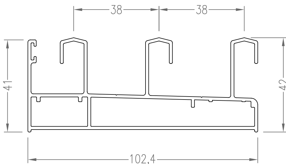
S285 Riel Triple 1.587 kg/m
