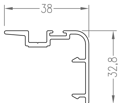
S283 Traslapo 0.398 kg/m
