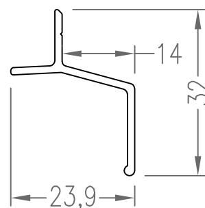
S286 Cortagotera 0.196 kg/m
